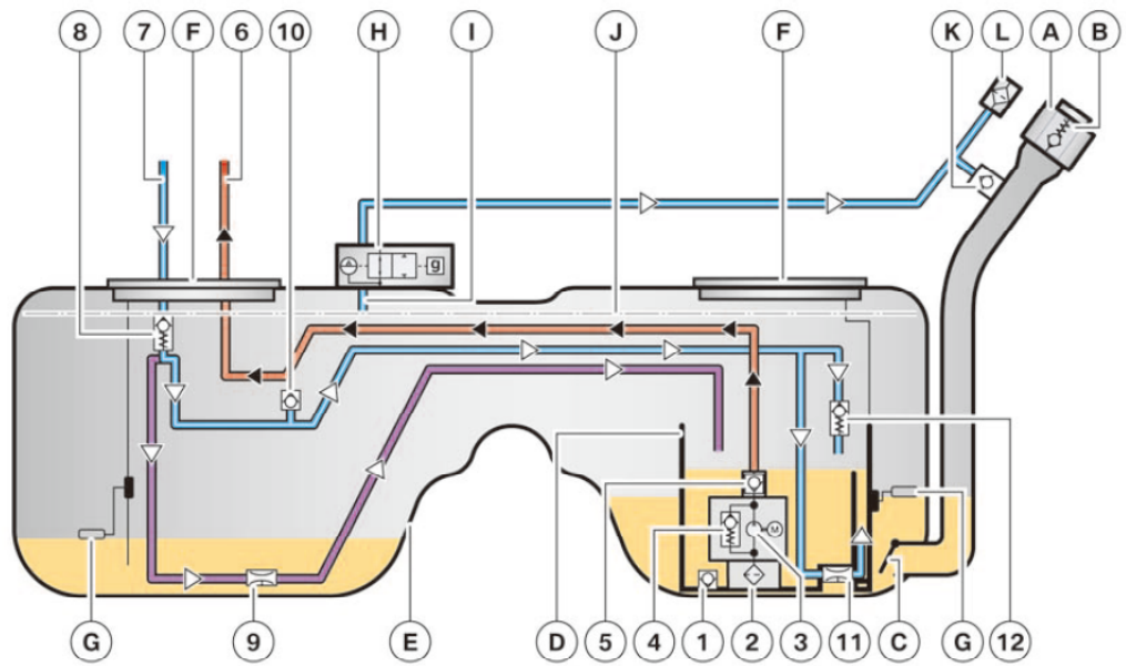
연료 시스템
