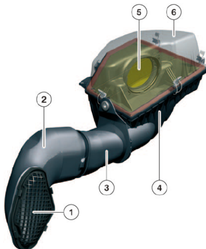
흡기 소음기
