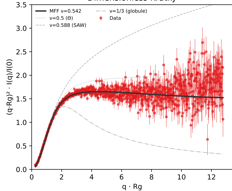
Dimensionless Kratky
