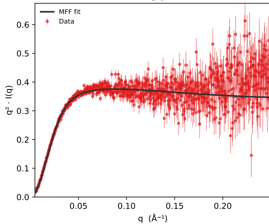
Kratky plot
