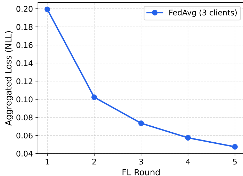
PyTorch MNIST — FL Convergence
