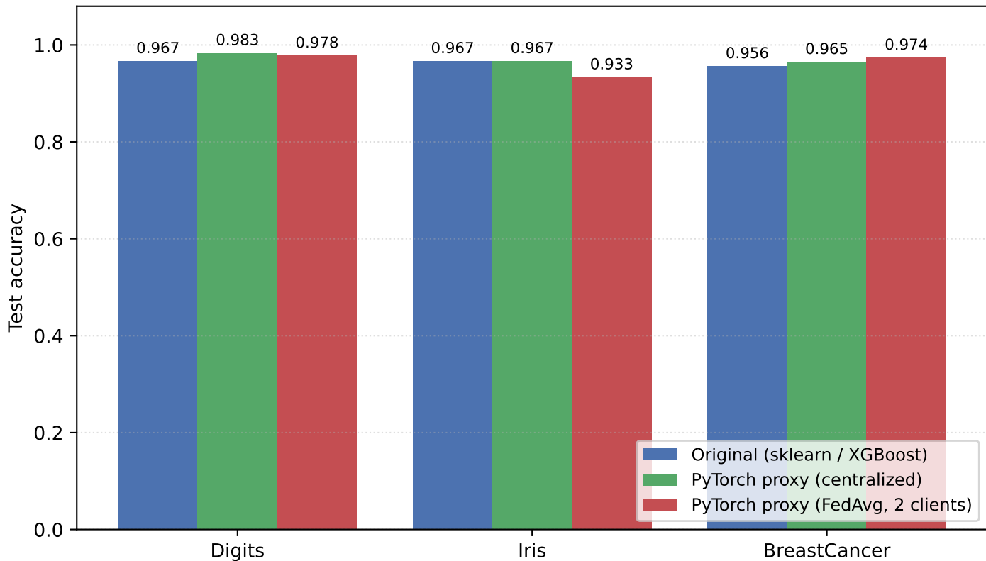
Non-DL benchmarks — original estimator vs PyTorch FL proxy
