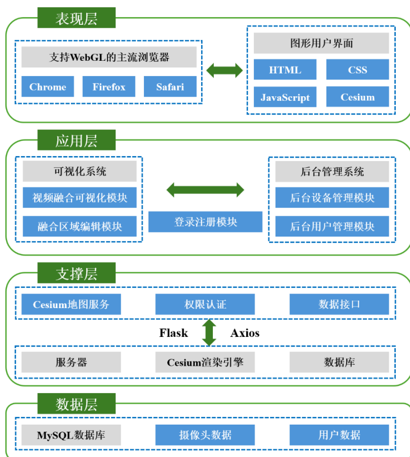
图 1. 系统架构图
