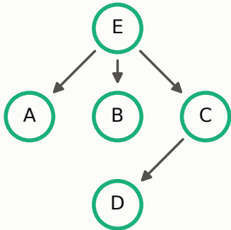
TRUE H*_2
