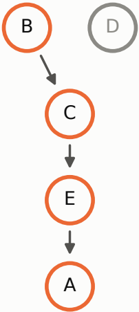
TRUE H*_1
