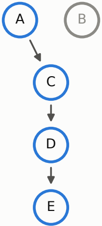
TRUE H*_0
