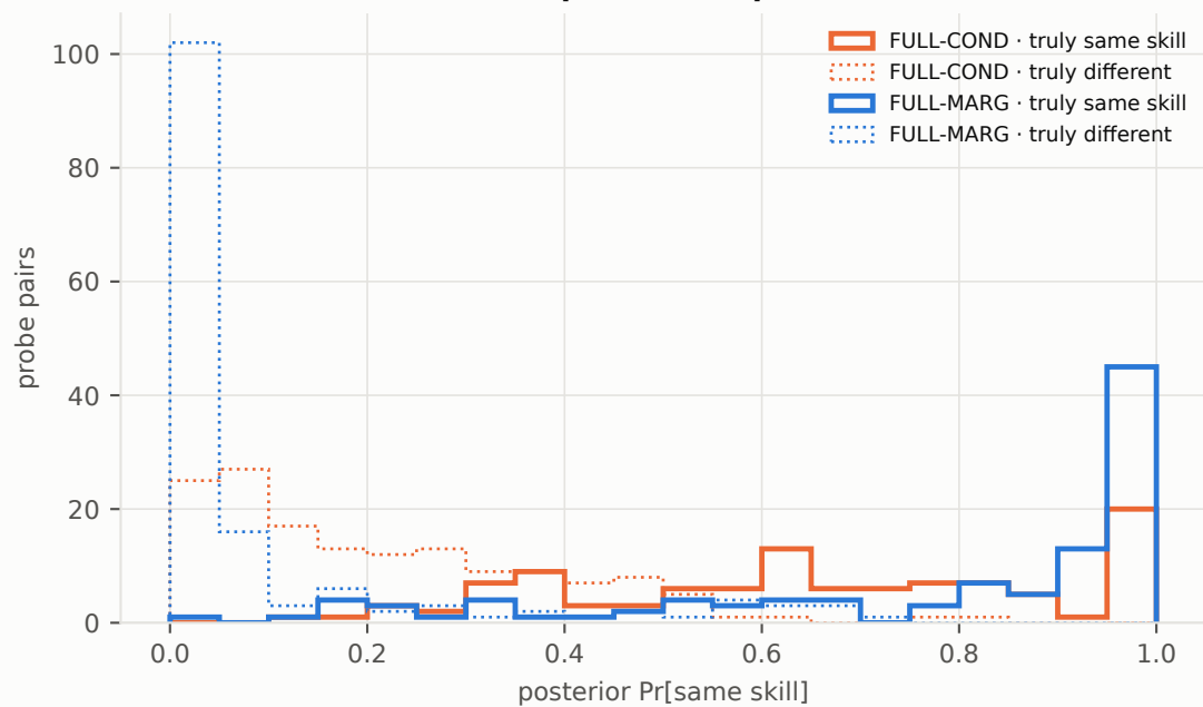
co-skill posterior separation
