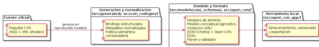
Figura 4.1: Arquitectura general de Open CVN organizada por capas, con el módulo del repositorio responsable de cada bloque.
