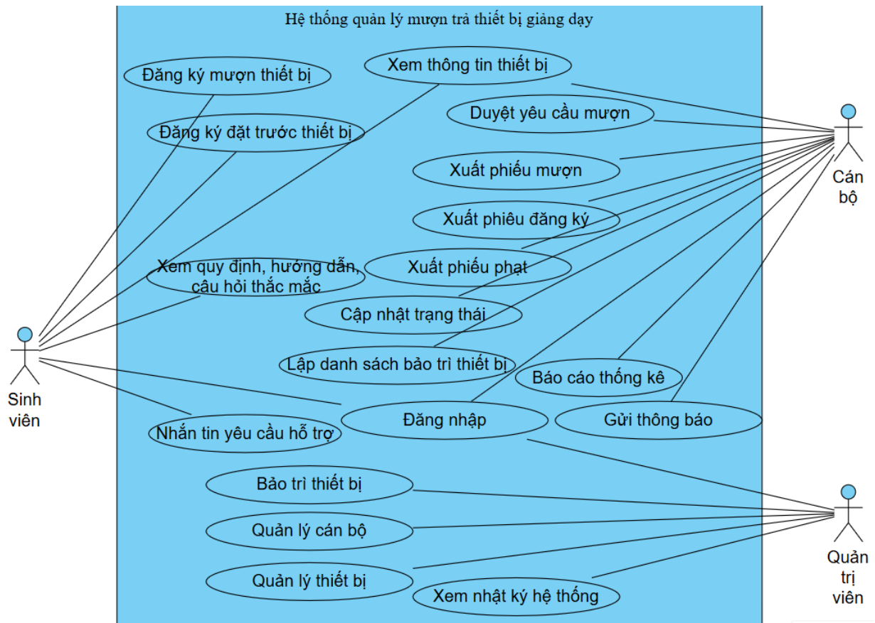
Hình 2.4 Sơ đồ Use case hệ thống
