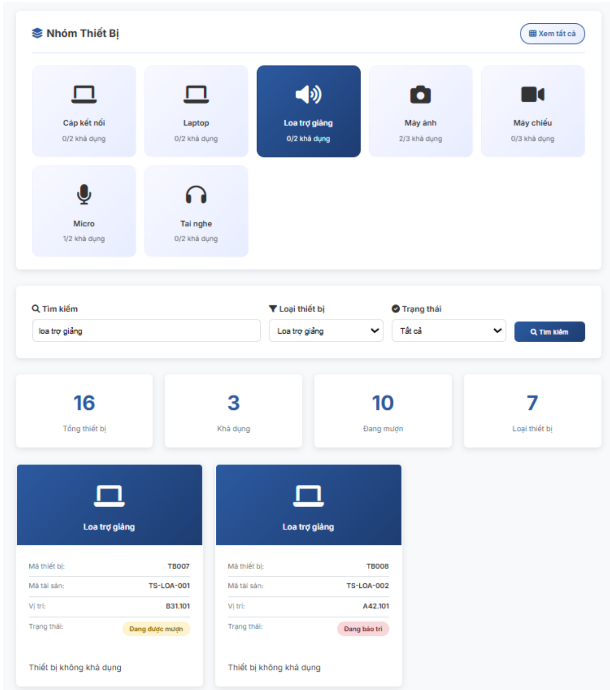
Hình 3.3 Giao diện chức năng tìm kiếm và lọc thông tin thiết bị
