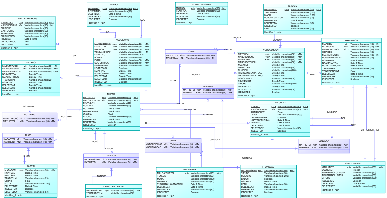
2.2.2. Mô hình dữ liệu mức logic và lược đồ CSDL
