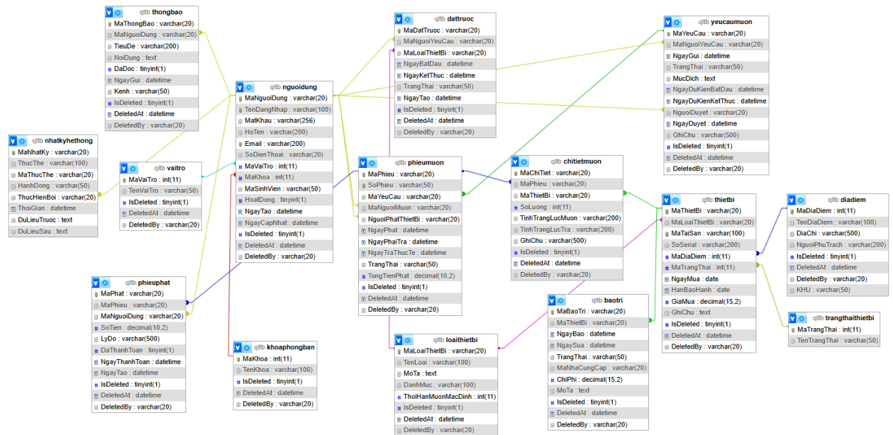
Hình 2.3 Lược đồ cơ sở dữ liệu
