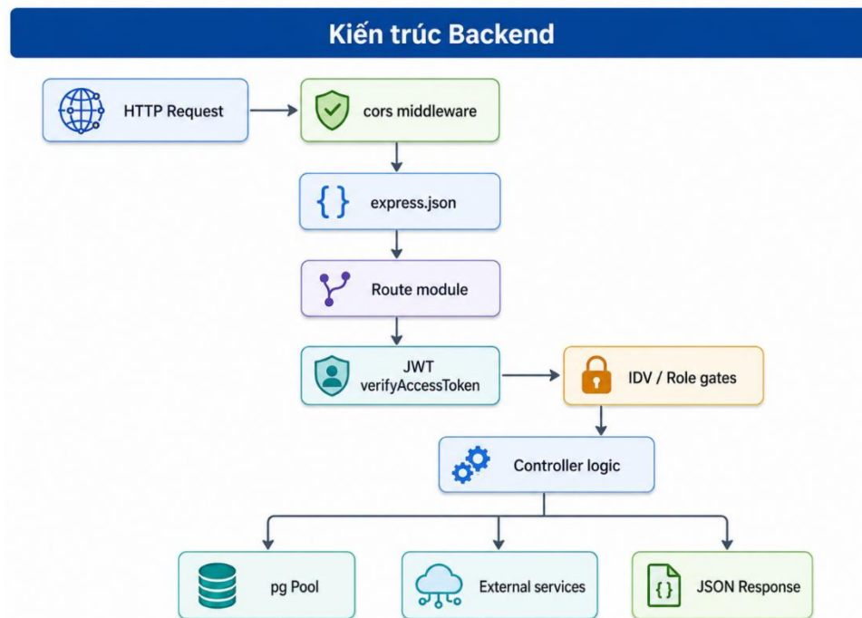
Hình 3.4 Sơ đồ kiến trúc back-end của hệ thống
