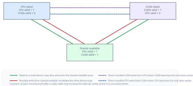
图 3.3: UVec 有效性状态机 (UVec validity-state machine)
