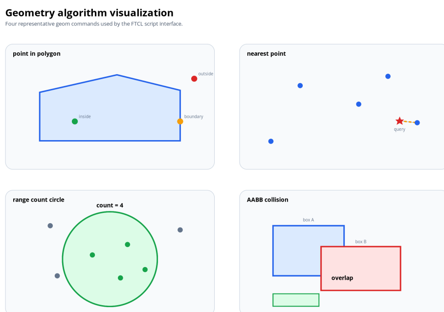
图 6.2: 代表性几何算法可视化 (Representative geometry algorithms)
