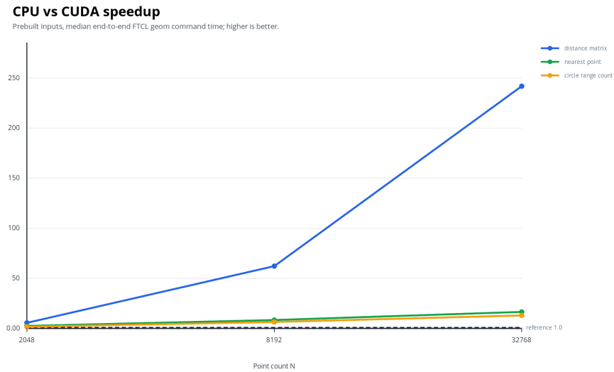
图 5.6: 批量几何算法的 CPU/CUDA speedup
