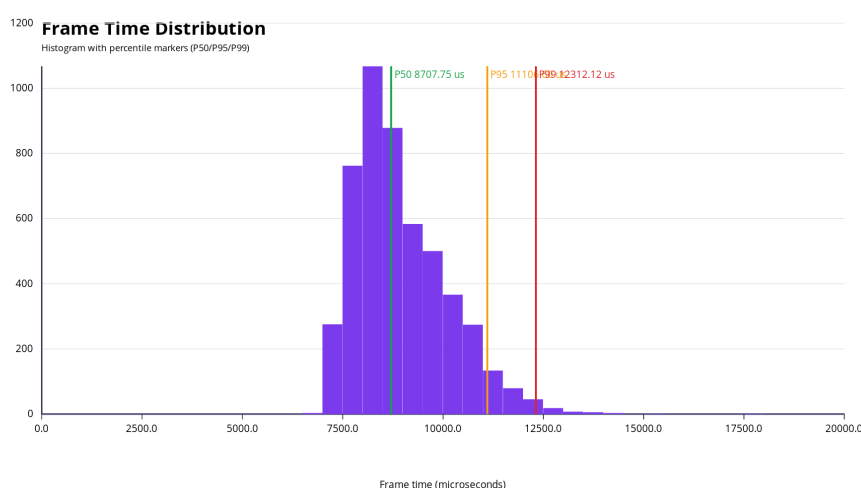
图 5.4: 类游戏 workload 的帧耗时分布 (Frame-time distribution)
