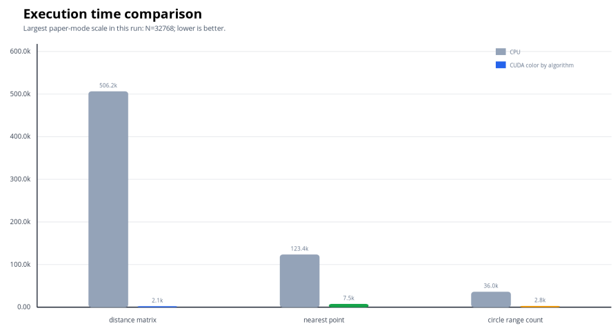
图 5.7: 最大测量规模下的执行时间对比 (Execution-time comparison)
