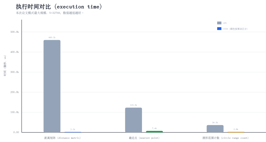
图 5.7: 最大测量规模下的执行时间对比 (Execution-time comparison)
