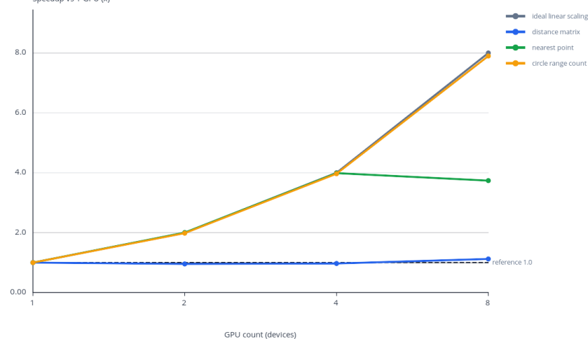
Figure 5.9: 1、2、4、8 张 A800 GPU 的 weak-scaling speedup
