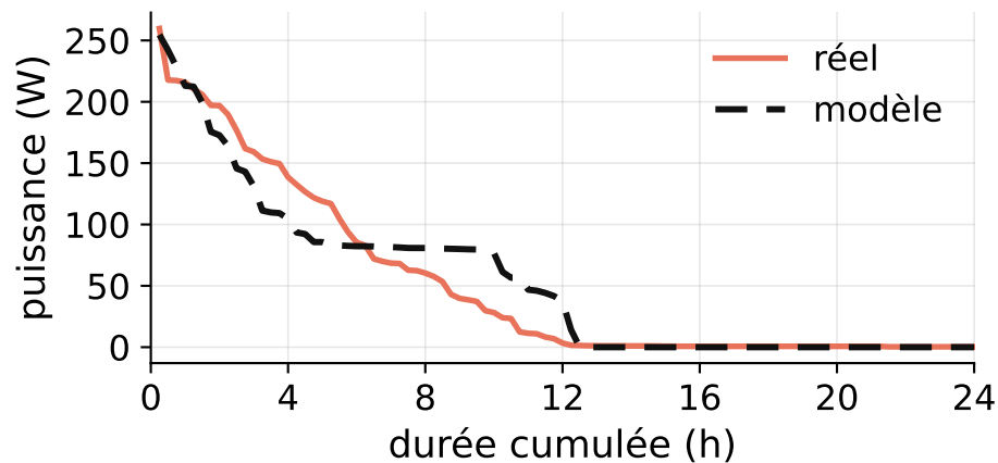
Courbe classée, LDC 8,1 %
