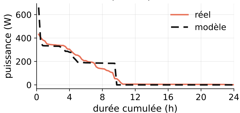
Courbe classée, LDC 8,4 %
