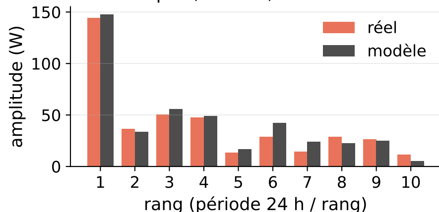
Harmoniques, FFT 13,5 %
