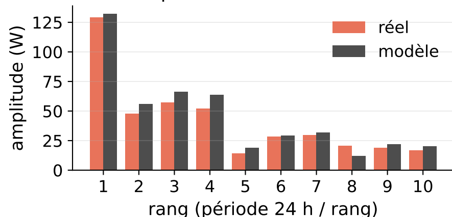
Harmoniques, FFT 10,3 %
