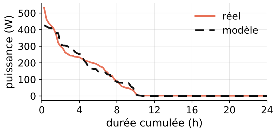
Courbe classée, LDC 3,9 %
