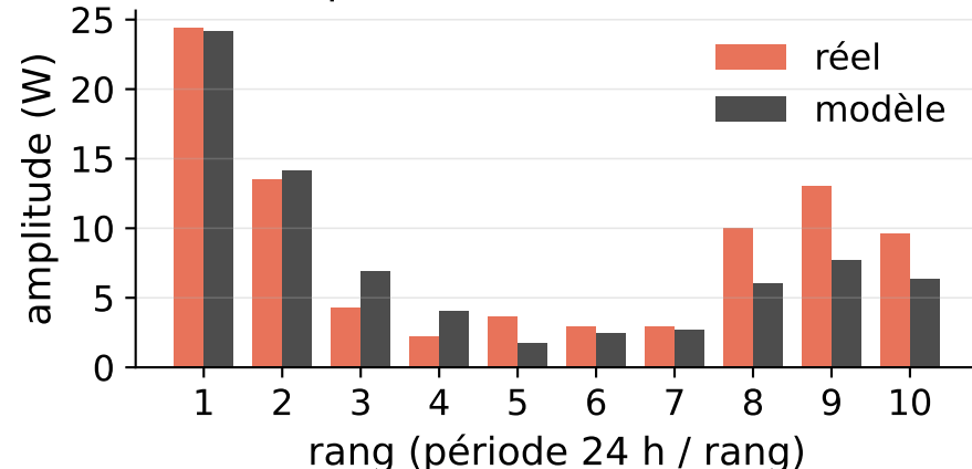
Harmoniques, FFT 18,1 %
