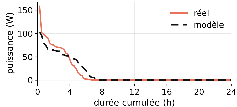
Courbe classée, LDC 6,1 %
