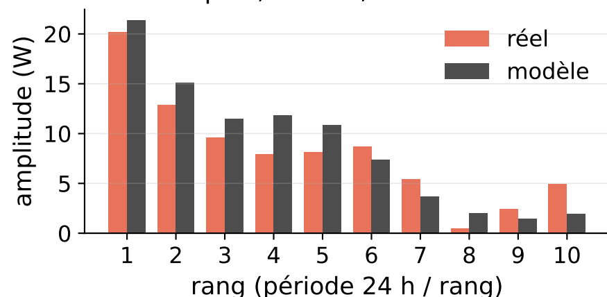
Harmoniques, FFT 16,0 %
