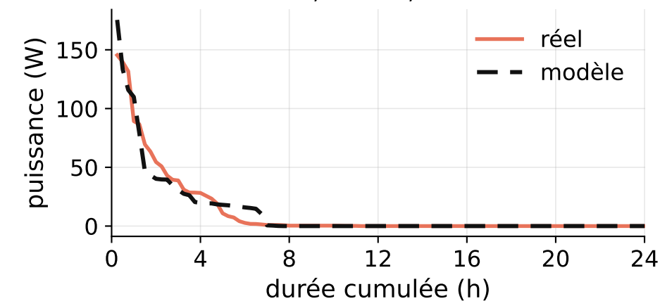
Courbe classée, LDC 4,6 %
