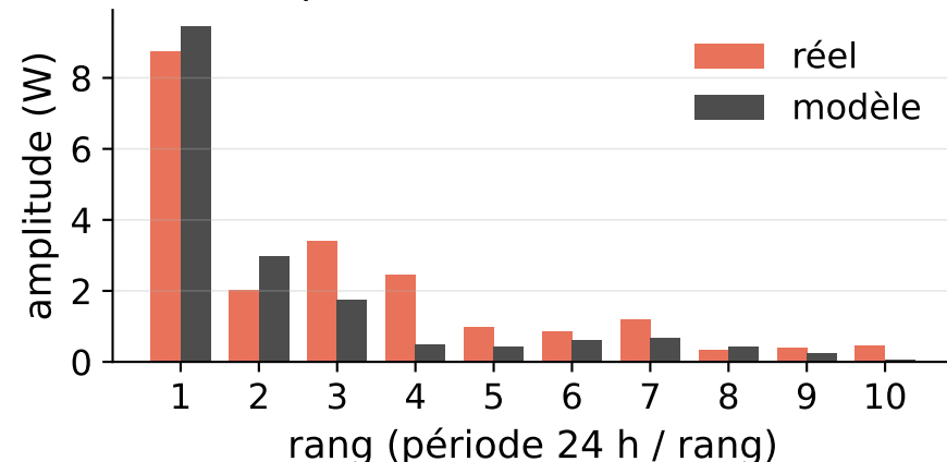
Harmoniques, FFT 28,2 %
