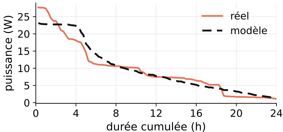
Courbe classée, LDC 7,3 %
