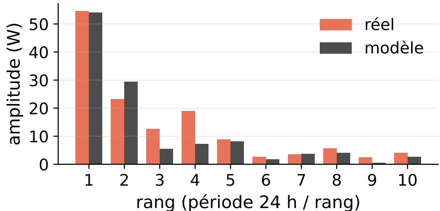
Harmoniques, FFT 21,7 %
