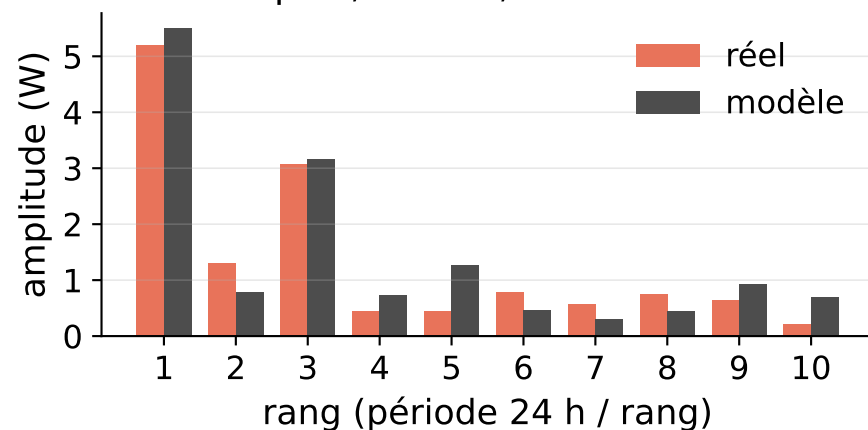
Harmoniques, FFT 20,0 %
