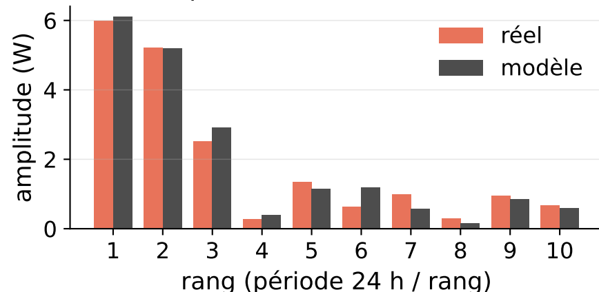
Harmoniques, FFT 11,4 %
