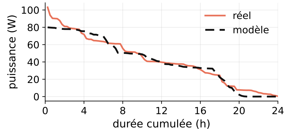
Courbe classée, LDC 5,2 %
