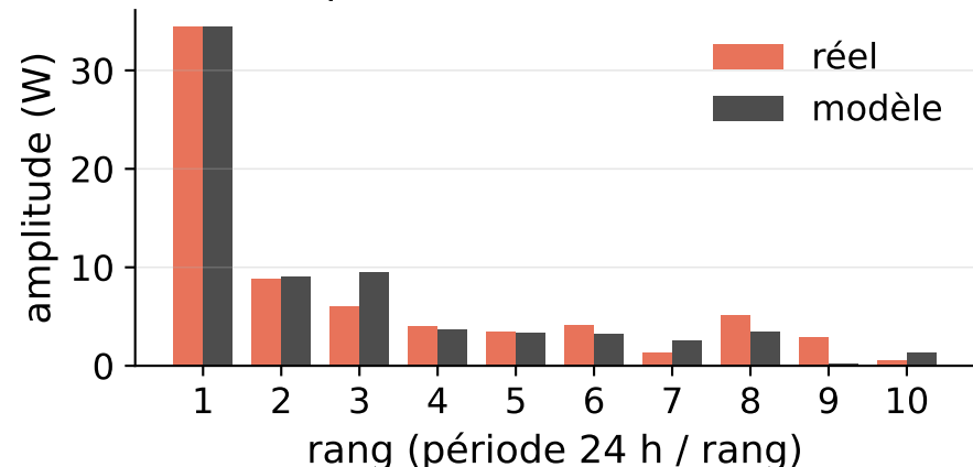
Harmoniques, FFT 21,9 %
