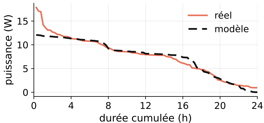
Courbe classée, LDC 6,7 %
