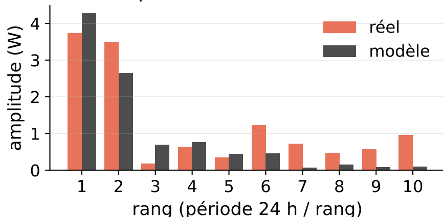
Harmoniques, FFT 43,9 %
