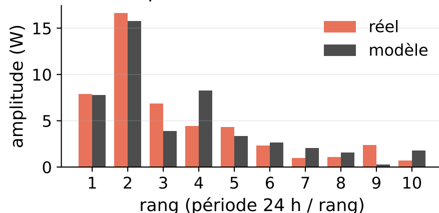
Harmoniques, FFT 26,9 %
