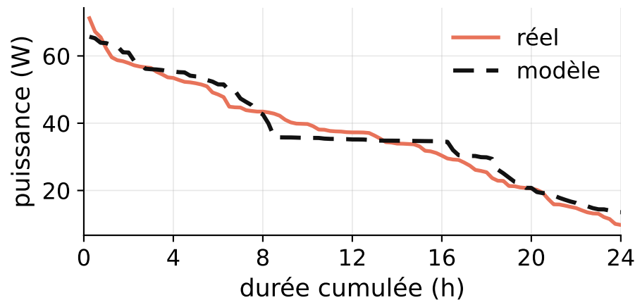
Courbe classée, LDC 4,6 %
