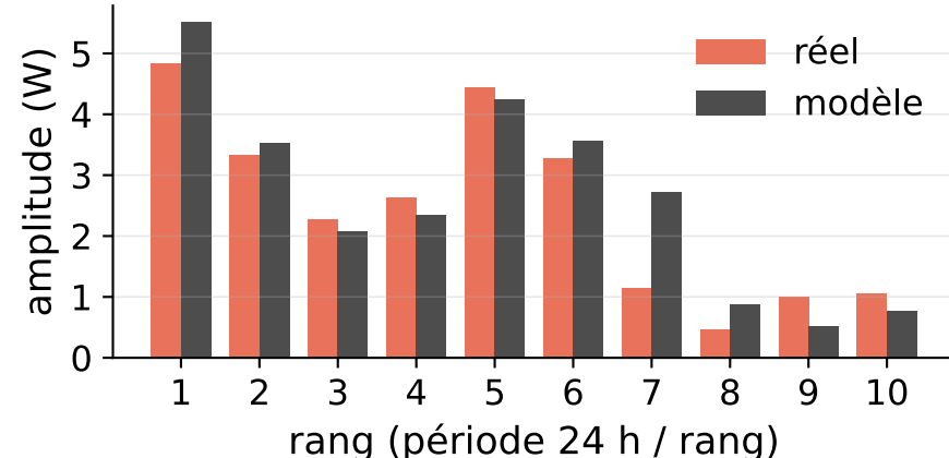
Harmoniques, FFT 17,6 %
