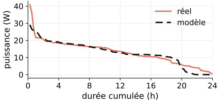
Courbe classée, LDC 5,5 %
