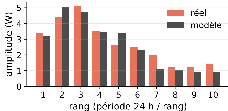
Harmoniques, FFT 18,8 %
