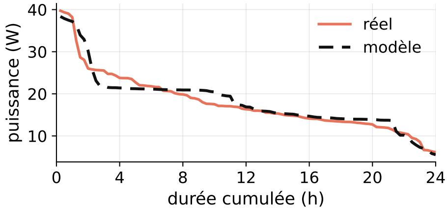
Courbe classée, LDC 5,2 %
