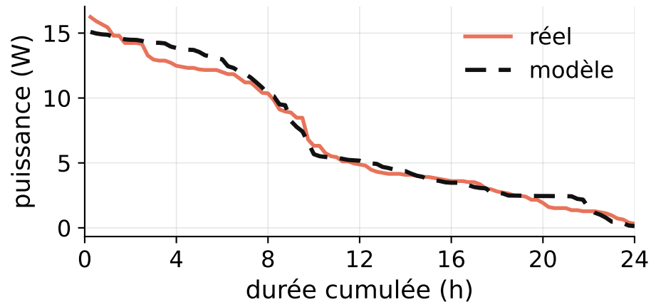
Courbe classée, LDC 4,0 %
