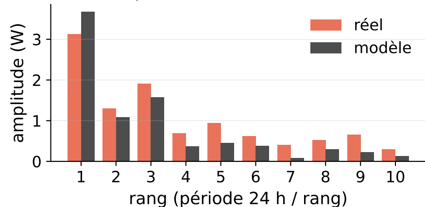
Harmoniques, FFT 31,5 %
