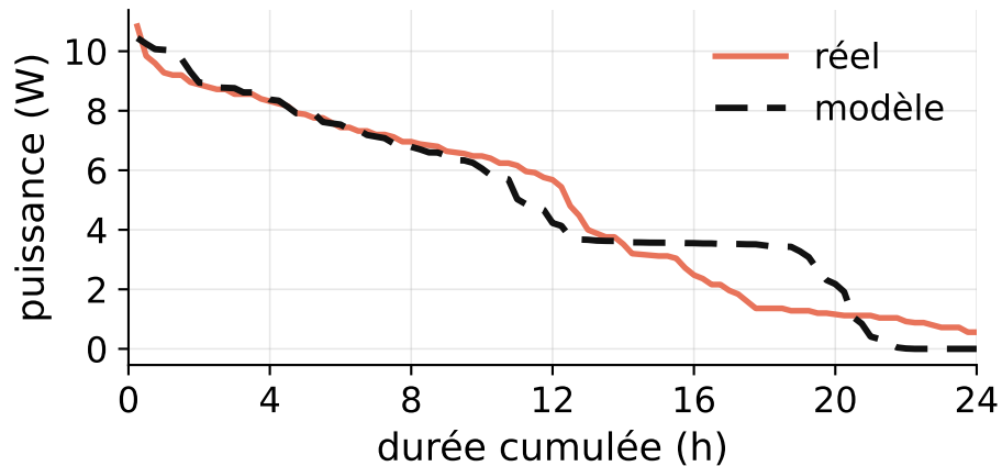
Courbe classée, LDC 8,6 %
