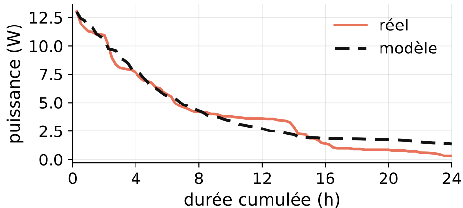
Courbe classée, LDC 5,4 %
