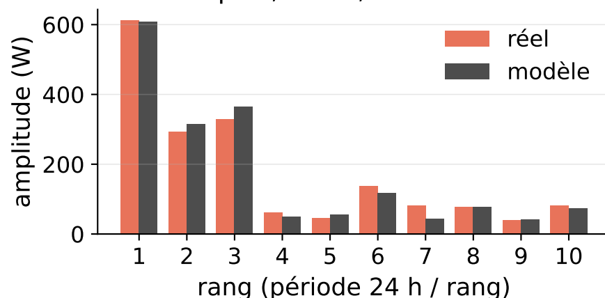
Harmoniques, FFT 8,4 %
