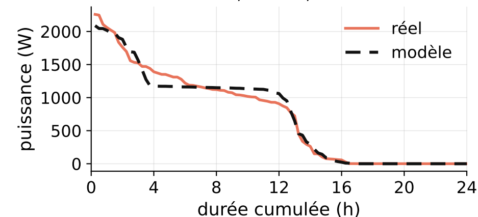
Courbe classée, LDC 4,0 %
