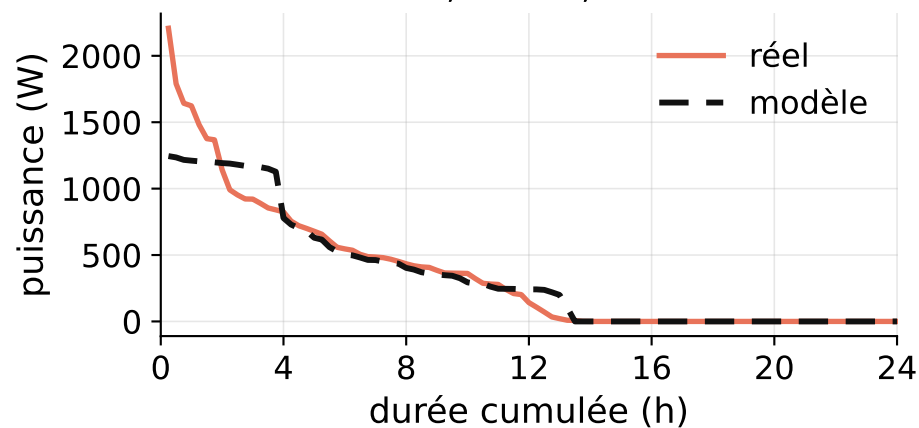
Courbe classée, LDC 7,1 %
