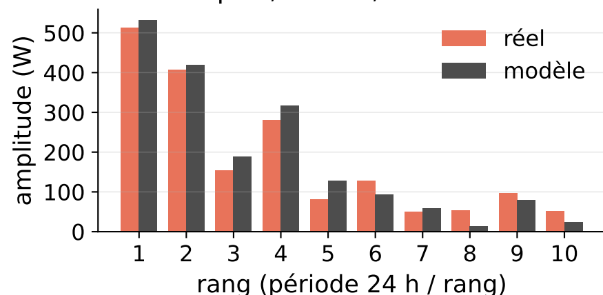
Harmoniques, FFT 22,7 %
