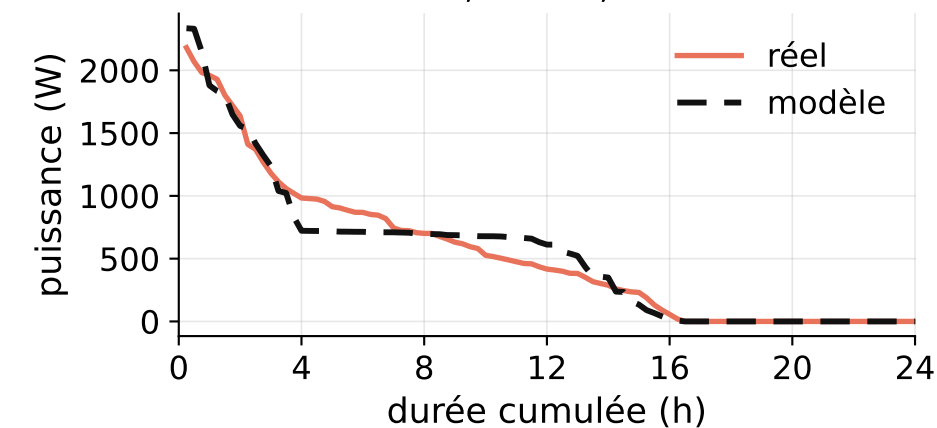
Courbe classée, LDC 5,0 %
