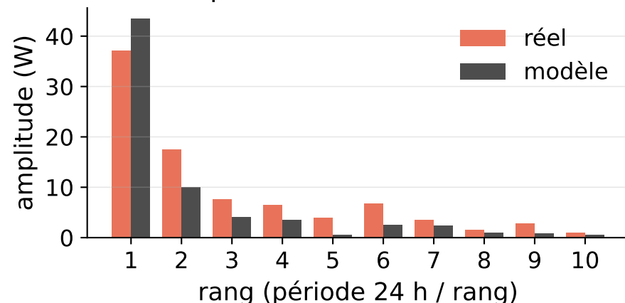
Harmoniques, FFT 24,3 %
