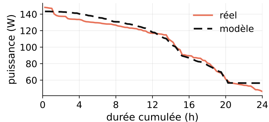
Courbe classée, LDC 4,6 %
