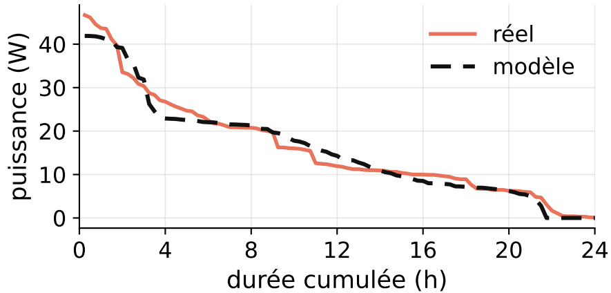
Courbe classée, LDC 4,1 %
