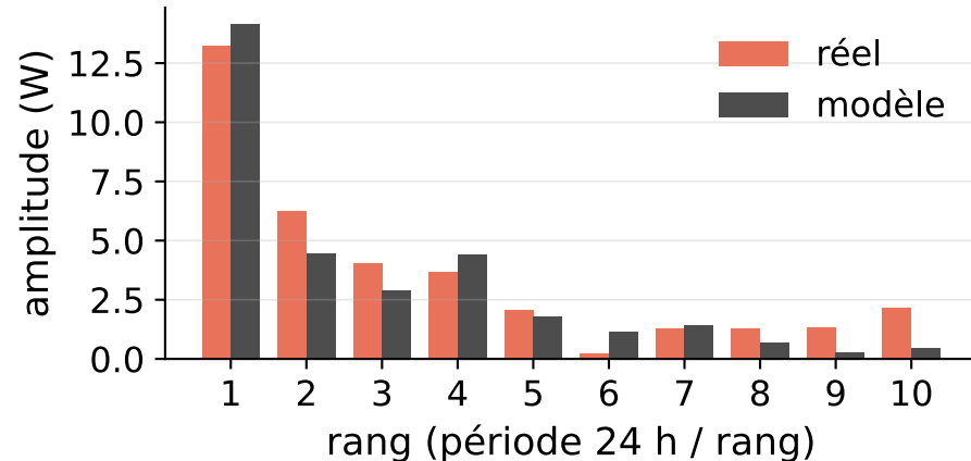
Harmoniques, FFT 22,5 %
