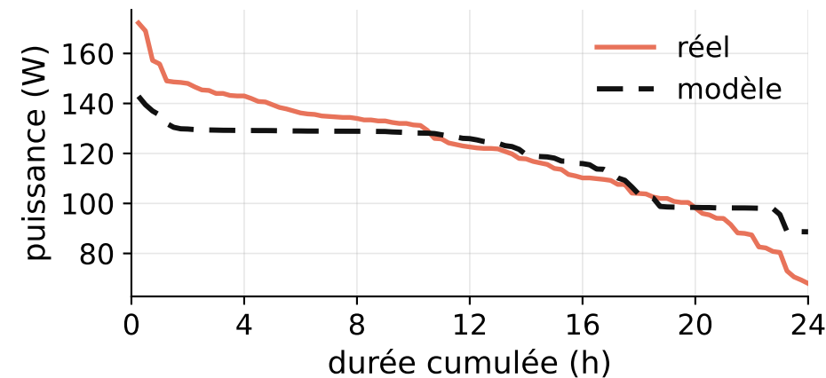
Courbe classée, LDC 9,8 %
