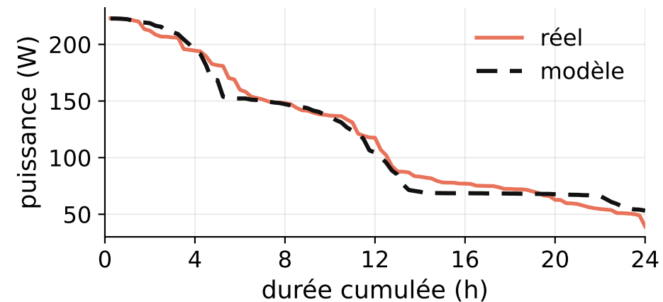
Courbe classée, LDC 4,3 %
