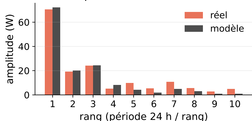
Harmoniques, FFT 26,5 %
