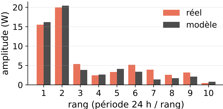
Harmoniques, FFT 12,1 %
