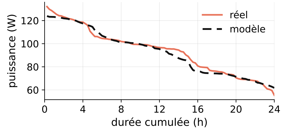
Courbe classée, LDC 4,2 %
