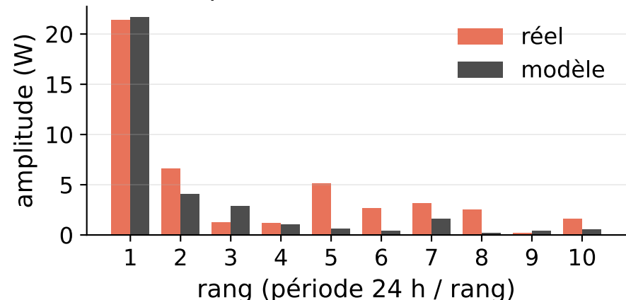
Harmoniques, FFT 28,4 %
