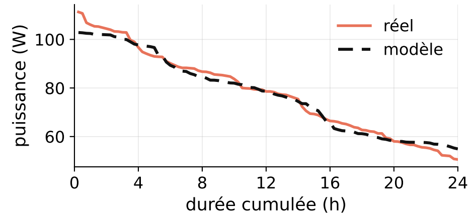
Courbe classée, LDC 4,1 %
