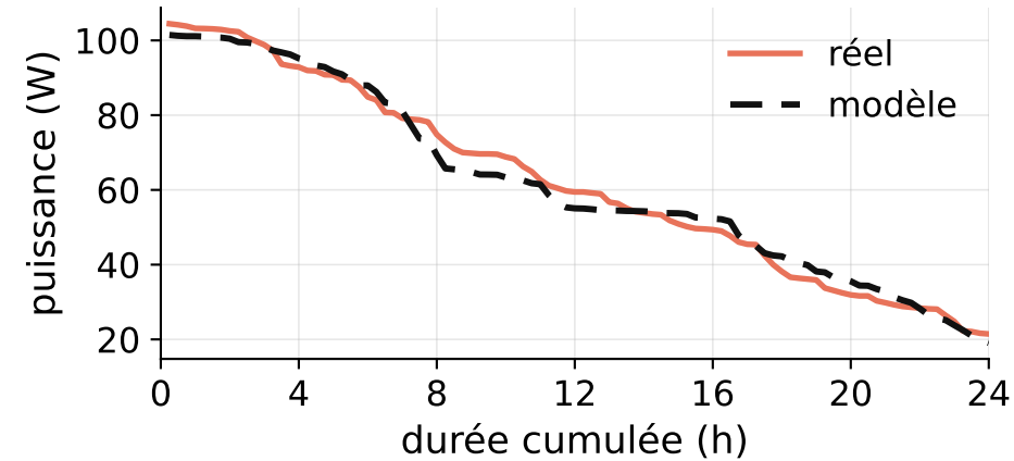
Courbe classée, LDC 3,7 %
