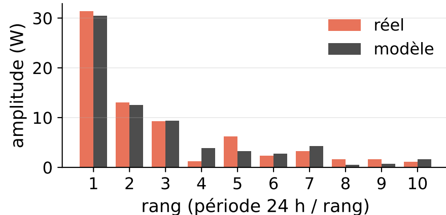
Harmoniques, FFT 19,4 %
