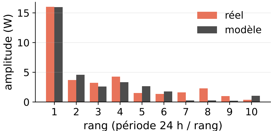
Harmoniques, FFT 28,3 %
