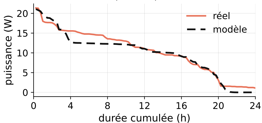
Courbe classée, LDC 6,2 %
