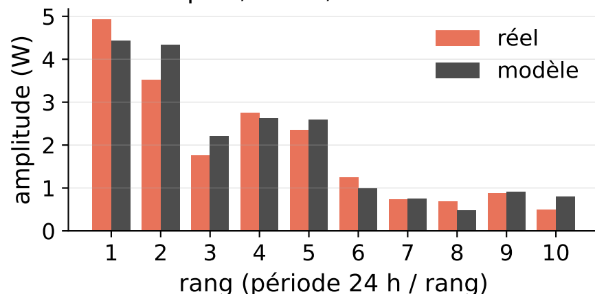
Harmoniques, FFT 9,9 %
