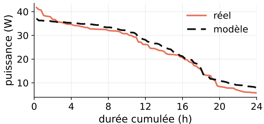
Courbe classée, LDC 5,0 %
