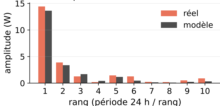
Harmoniques, FFT 14,5 %
