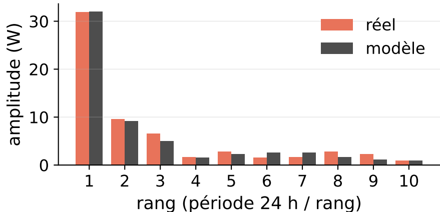
Harmoniques, FFT 10,2 %
