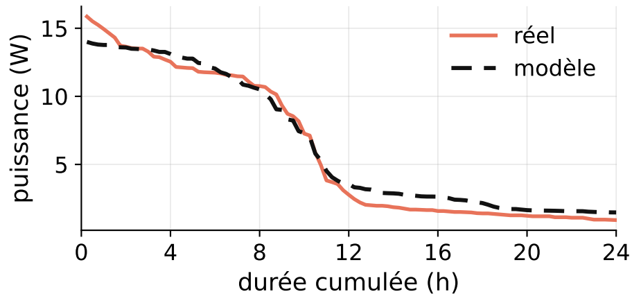
Courbe classée, LDC 4,8 %
