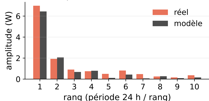
Harmoniques, FFT 21,7 %
