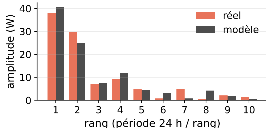
Harmoniques, FFT 25,1 %
