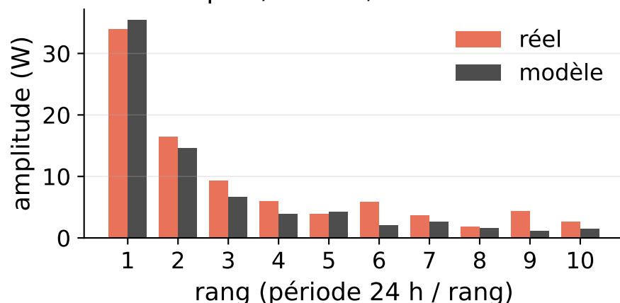
Harmoniques, FFT 20,9 %
