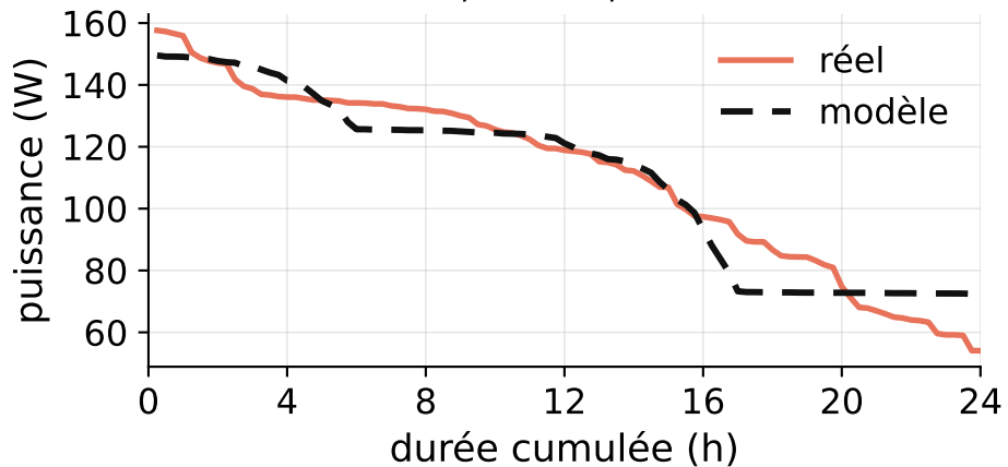
Courbe classée, LDC 7,6 %
