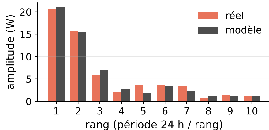
Harmoniques, FFT 10,1 %
