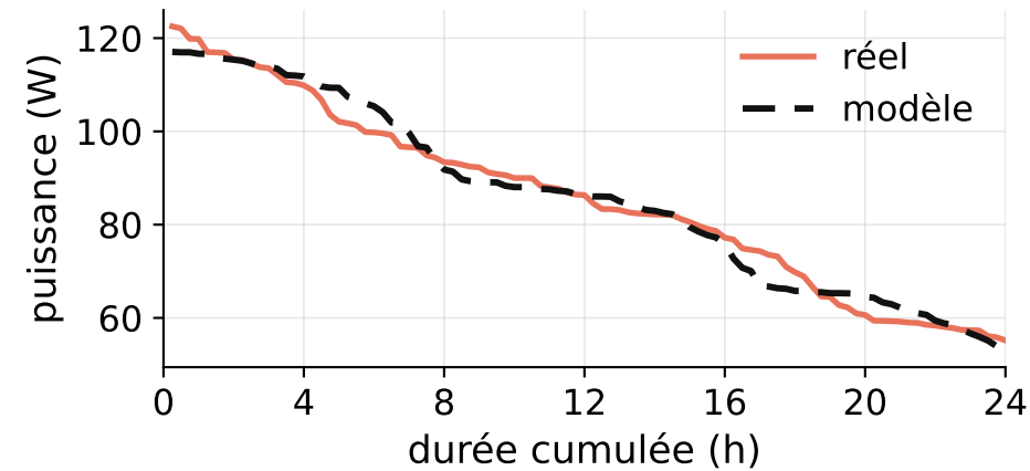
Courbe classée, LDC 4,5 %
